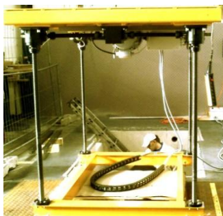
Spindelhubanlage
